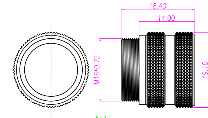
NUT
